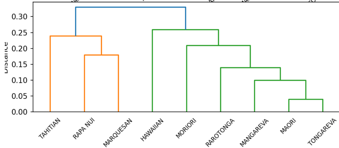
Дальний сосед (полное связывание)
